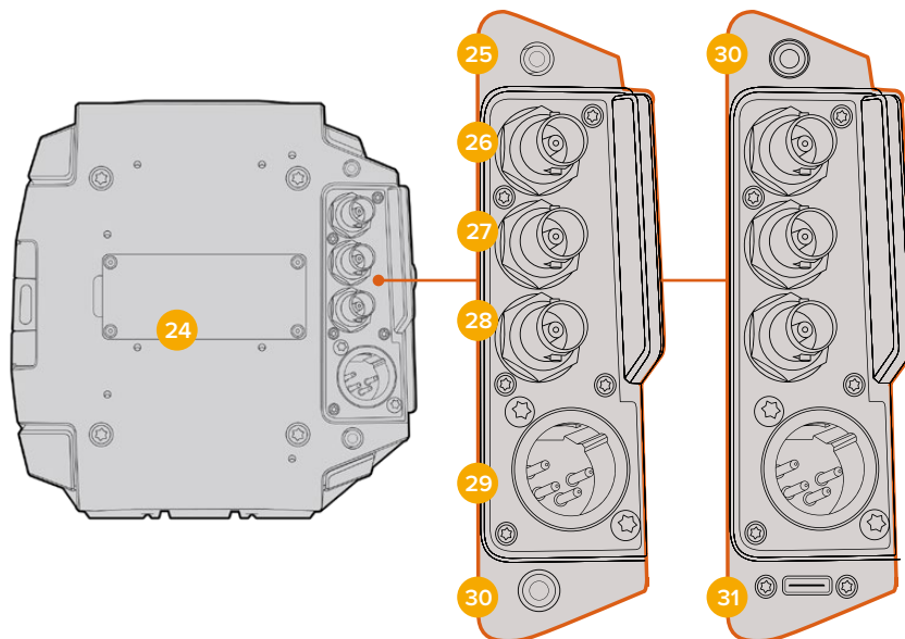
URSA Mini Pro 4.6K G2, URSA Mini Pro 4.6K, URSA Mini Pro 12K and URSA Mini 4.6K and URSA Mini 4K URSA Mini Pro 12K OLPF
